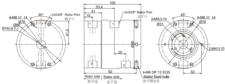
4进4出 G3/8"牙
