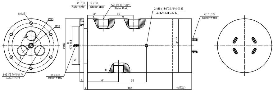
DAFH300-05气电一体 尺寸图 ▼
