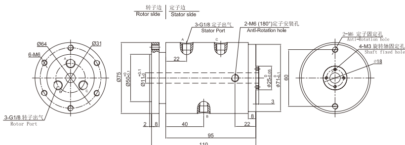
DA PH300-02纯气尺寸图 ▼
