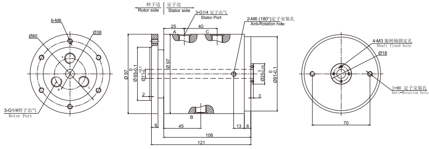
DAFH300-03纯气 尺寸图 ▼
