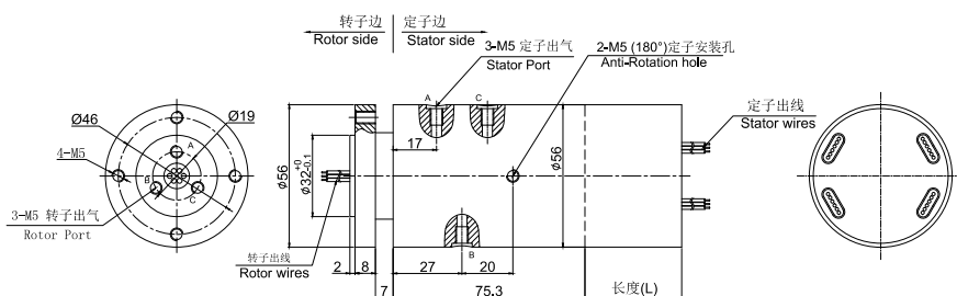
DA PH300-01气电一体尺寸图 ▼
