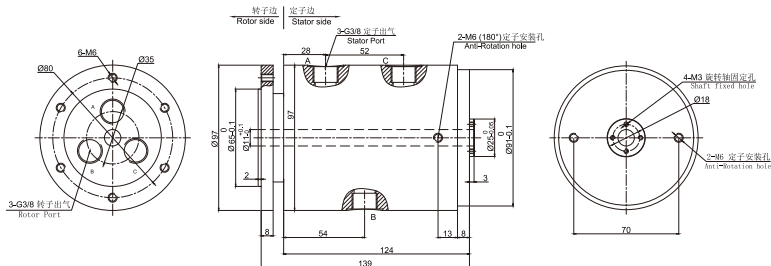
3进3出, G3/8接头 DAPH300-04 尺寸图
