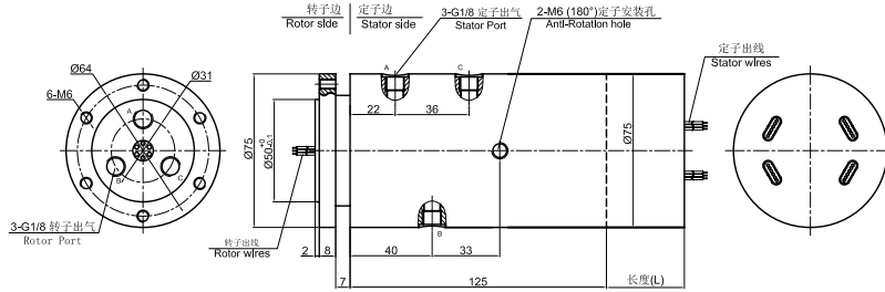
DAFH300-02气电一体 尺寸图 ▼
