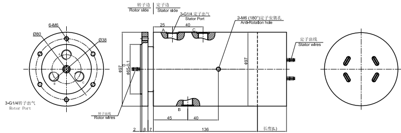
DAFH300-03气电一体 尺寸图 ▼
