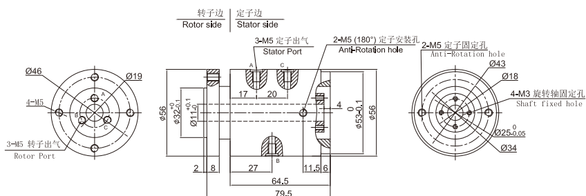
DA PH300-01纯气尺寸图 ▼
