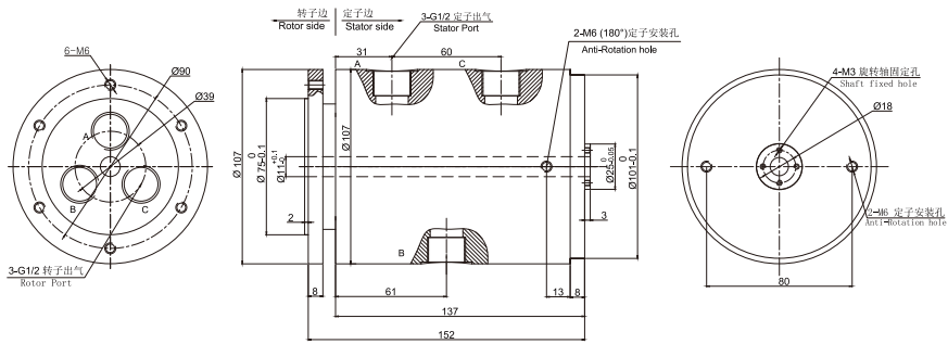
DAFH300-05气电一体 尺寸图 ▼
