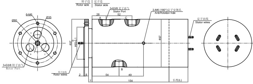
DAFH300-04气电一体 尺寸图 ▼
