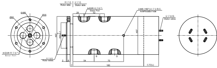
DAPH400-04气电一体 尺寸图 ▼
