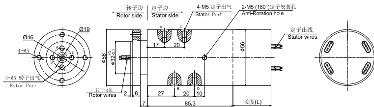
4进4出, G1/8接头 DAPH400-02 尺寸图
