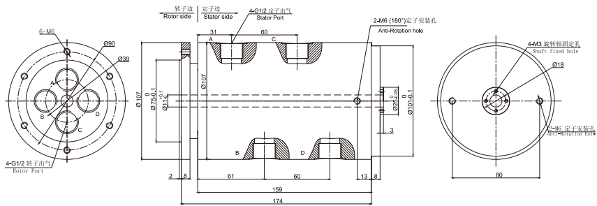
DAPH400-05纯气 尺寸图 ▼
