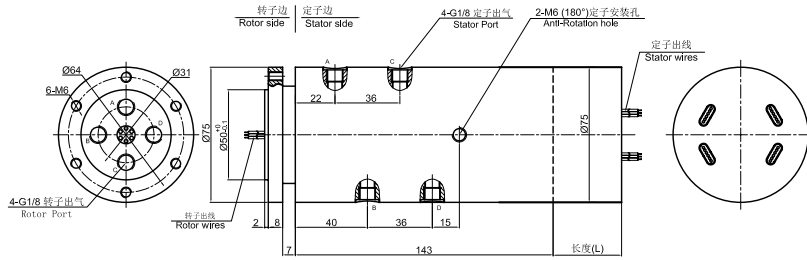
DAH400-02气电一体 尺寸图 ▼
