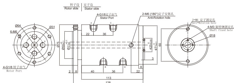
DAFH400-02纯气尺寸图 ▼
