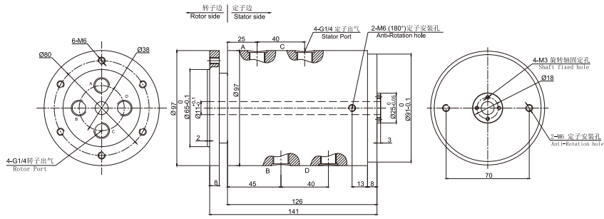
DAH400-03气电一体 尺寸图 ▼
