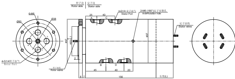
4进4出, G3/8接头 DAH400-04 尺寸图
