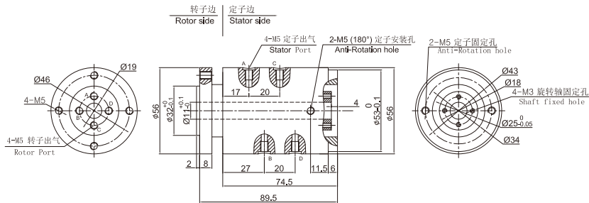
DAFH400-01气电一体尺寸图 ▼
