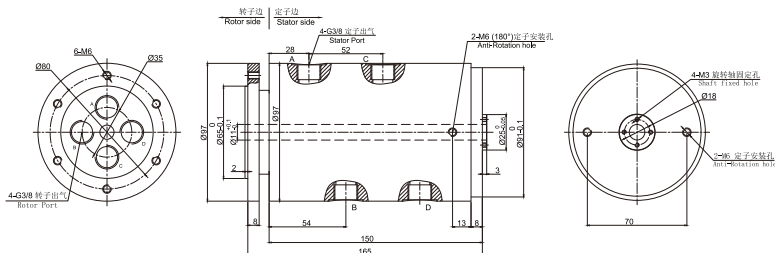
DAH400-04纯气 尺寸图 ▼
