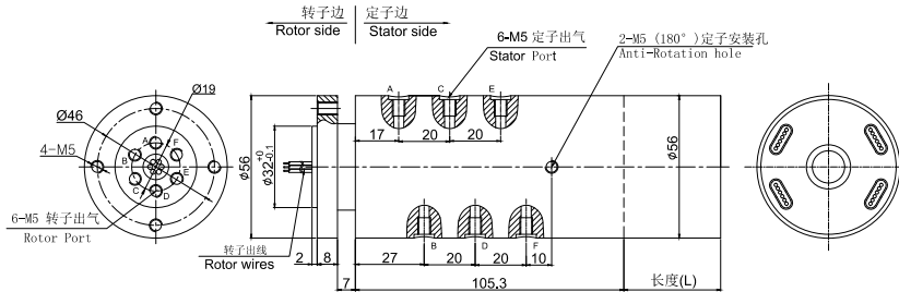
DAFH600-01气电一体 尺寸图 ▼
