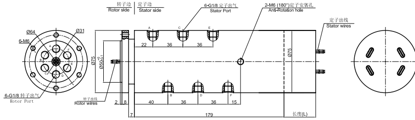
DAFH600-02气电一体 尺寸图 ▼
