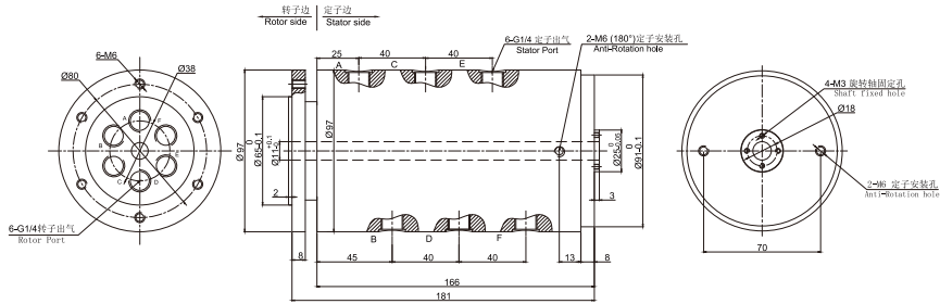
DAFH600-03纯气 尺寸图 ▼
