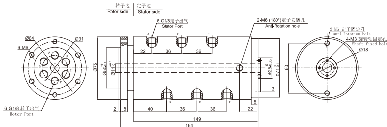
DAFH600-02纯气 尺寸图 ▼
