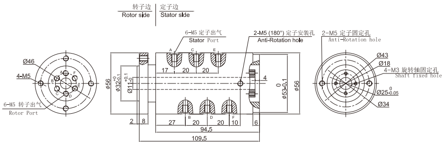
DAFH600-01纯气 尺寸图 ▼
