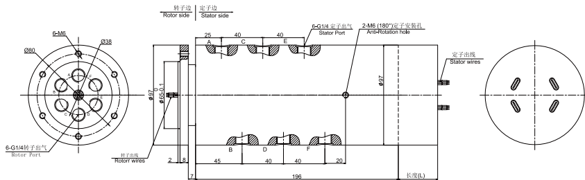
DAFH600-03气电一体 尺寸图 ▼
